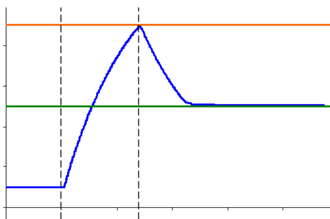
Рисунок 3 Процесс автонастройки и переход в режим автомат
