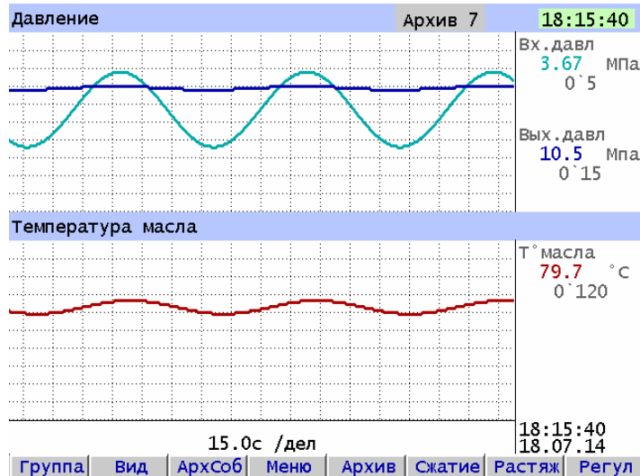
Рисунок 6.2 – Пример отображения несжатых графиков измерений двух групп каналов на двух лентах.
