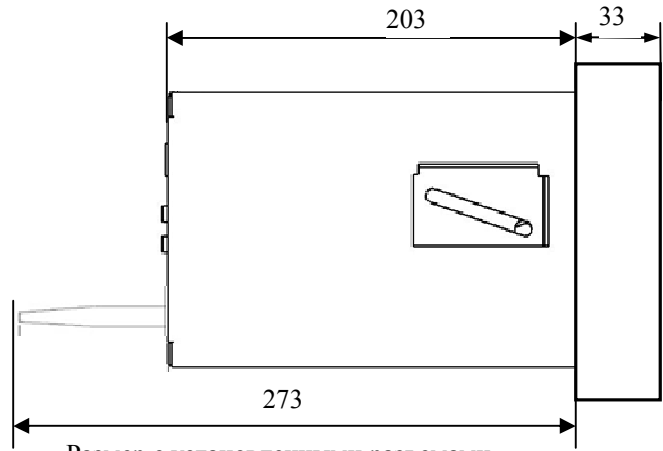
Размер с установленными разъемами
