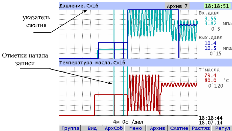
Рисунок 6.3 – Пример отображения сжатых графиков измерений двух групп каналов на двух лентах.
