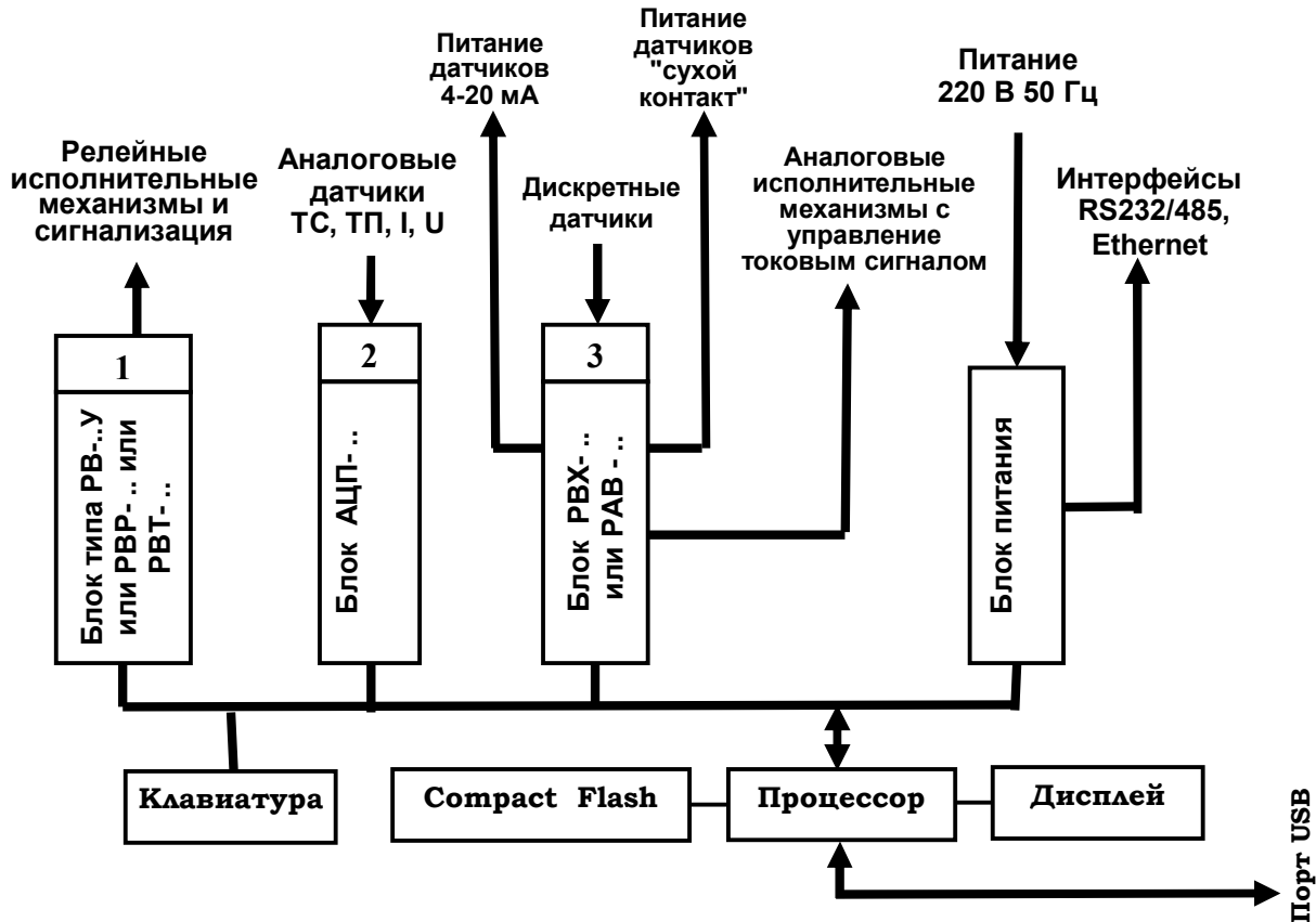
Рисунок 3.1 - Структурная схема прибора
