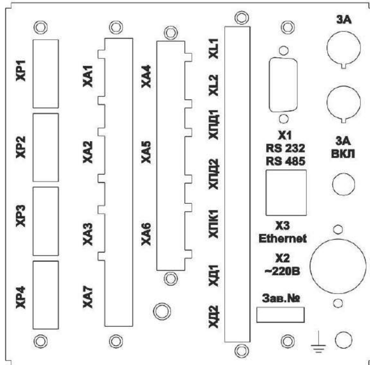
Прибор с аналоговыми выходами (с блоками РВ (РВР, РВТ), АЦП и РАВ)
