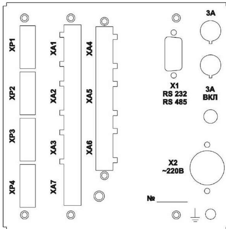
Прибор без аналоговых выходов, релейных входов и Ethernet (с блоками АЦП и РВ (РВР, РВТ))
