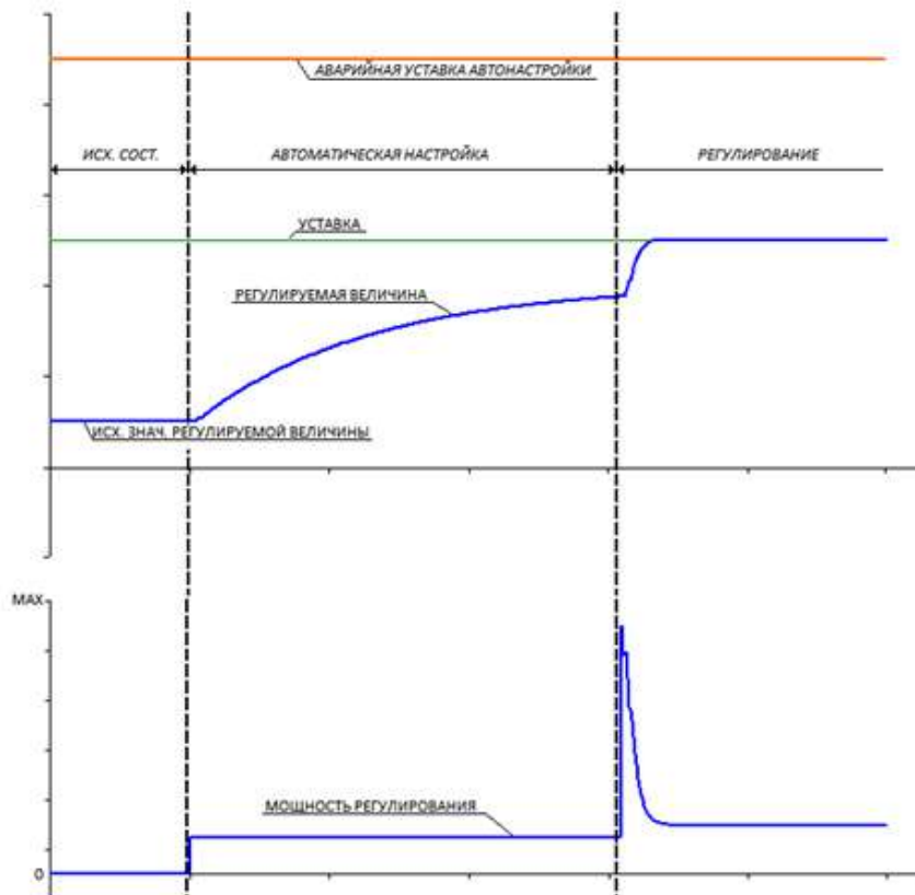
Рисунок 1 - Процесс автонастройки и переход в режим автомат
