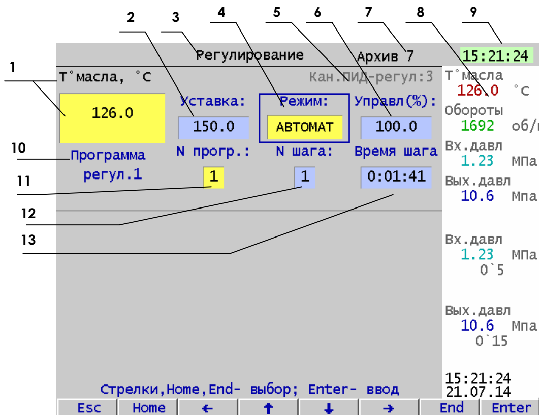
Рисунок 6.12 – Пример окна управления регуляторами
