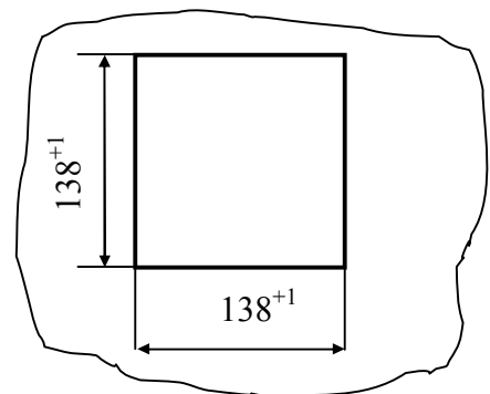
Вырез в щите
